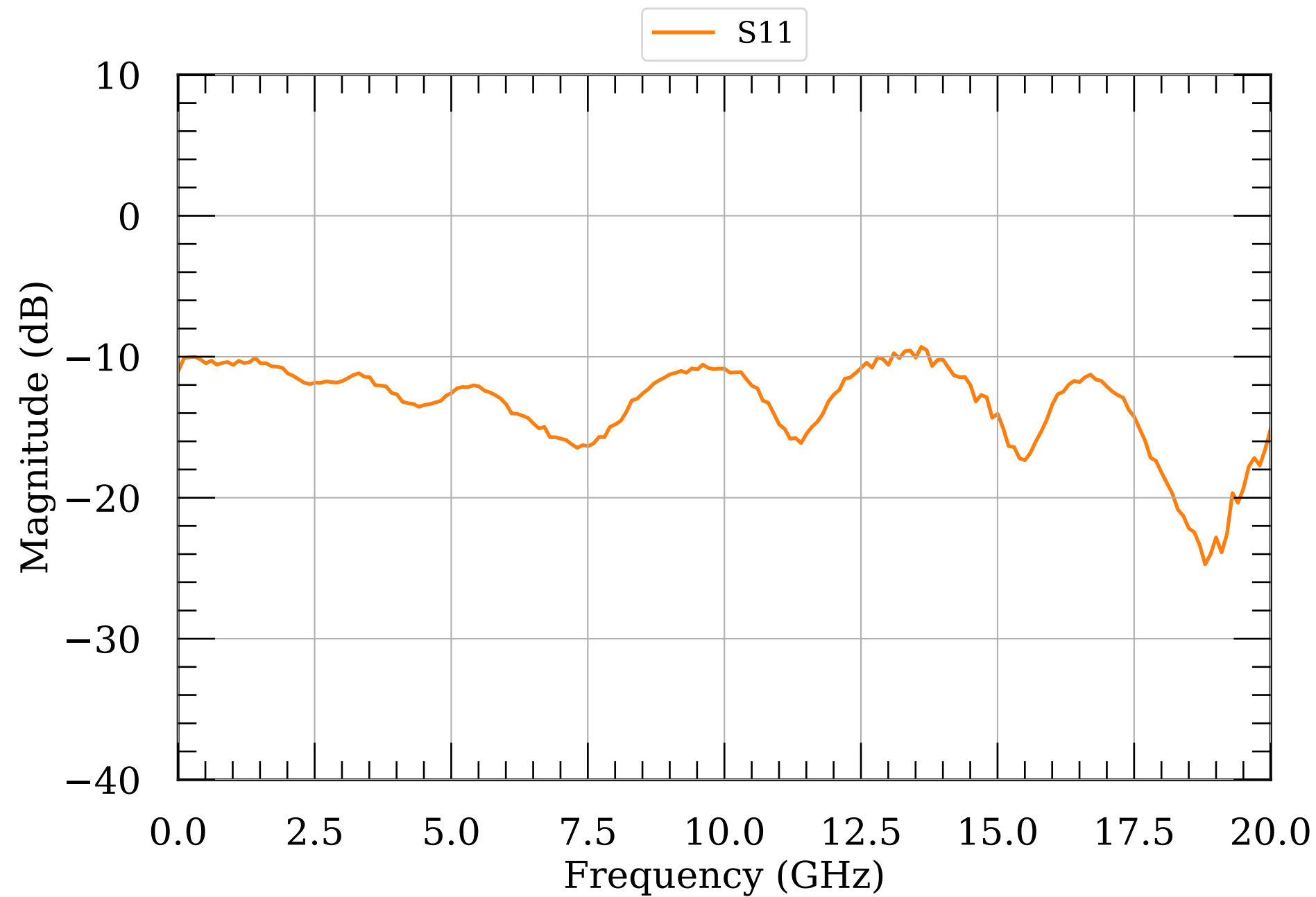
LNA S-params module035
